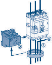
VigiPacT modülü ComPacT NSX
